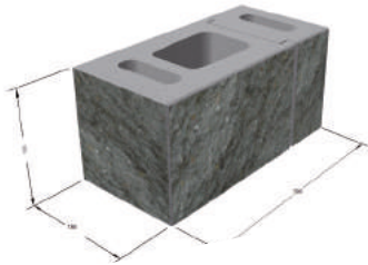
Pustak słupkowy łupany czterostronnie 2- elementowy słupek typu B A-PO 19/4
